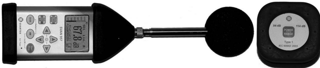
21 pav. SVAN 957 Triukšmo ir vibracijos matuoklis.
