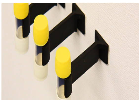
5 pav. amoniako (NH 3 ) pasyvus serbentas
